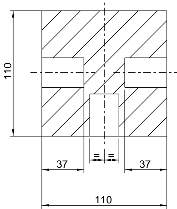
Coupe B-B
